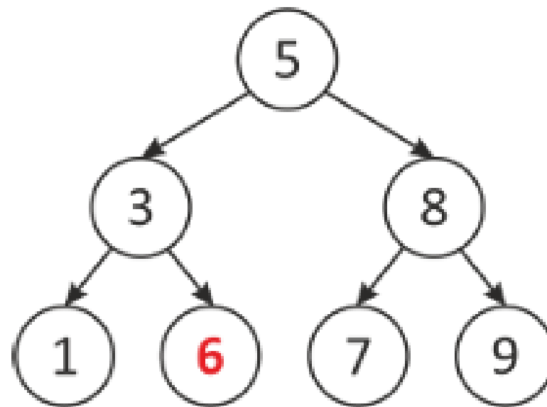
Не является деревом поиска
